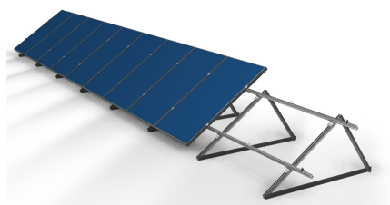
Система крепления «Актив» Материал - алюминиевый сплав АД31 Т5, (6061Т5) Метиз – нержавейка А2;
